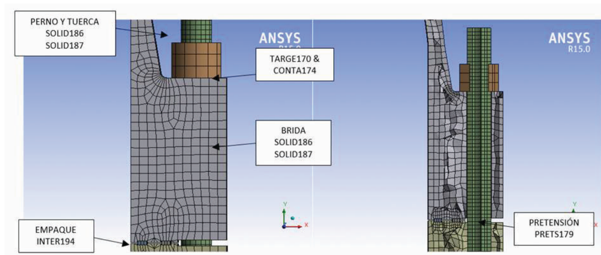
Fig. 4. Generación de malla del modelo.
