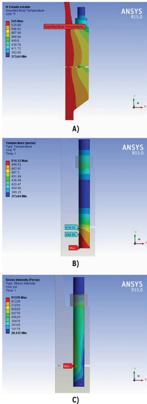
Fig. 5. Resultados del estado estable: A) Distribución de temperatura en modelo, B) Distribución de temperatura en el perno C) Intensidad de esfuerzo en el perno.
