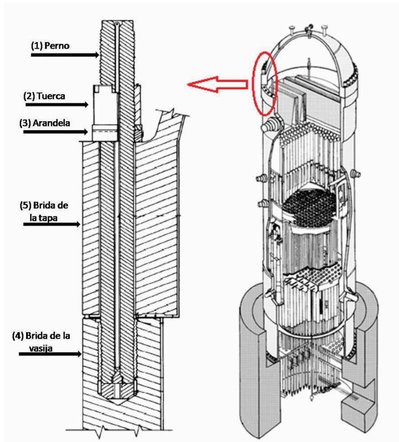
Fig. 1. Conjunto de cierre de la vasija.
